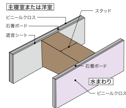
■水まわり間仕切り壁断面図(施工例)
