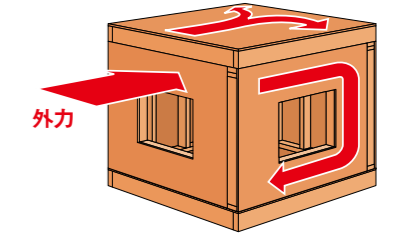
■ダイヤフラムで構成されたモノコック構造（概念図）
