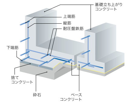
■基礎施工例(概念図)
