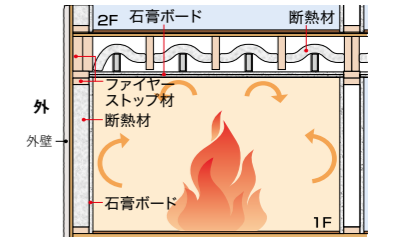
■ファイヤーストップ構造例（概念図）
