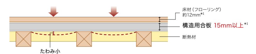
■1階床施工例（概念図）
